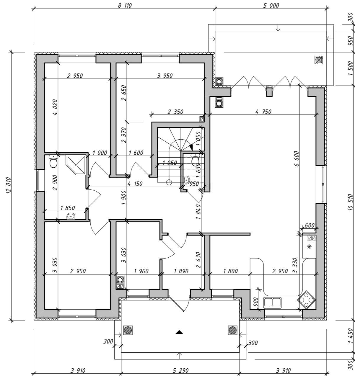
План 1-го этажа
